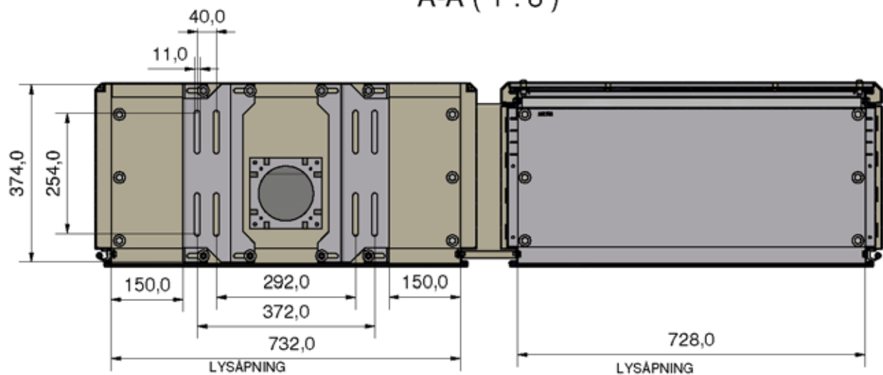
A-A (1 : 8)
