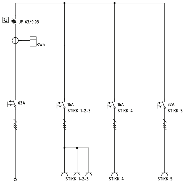
71012 HS 63A 00113-R 230V
