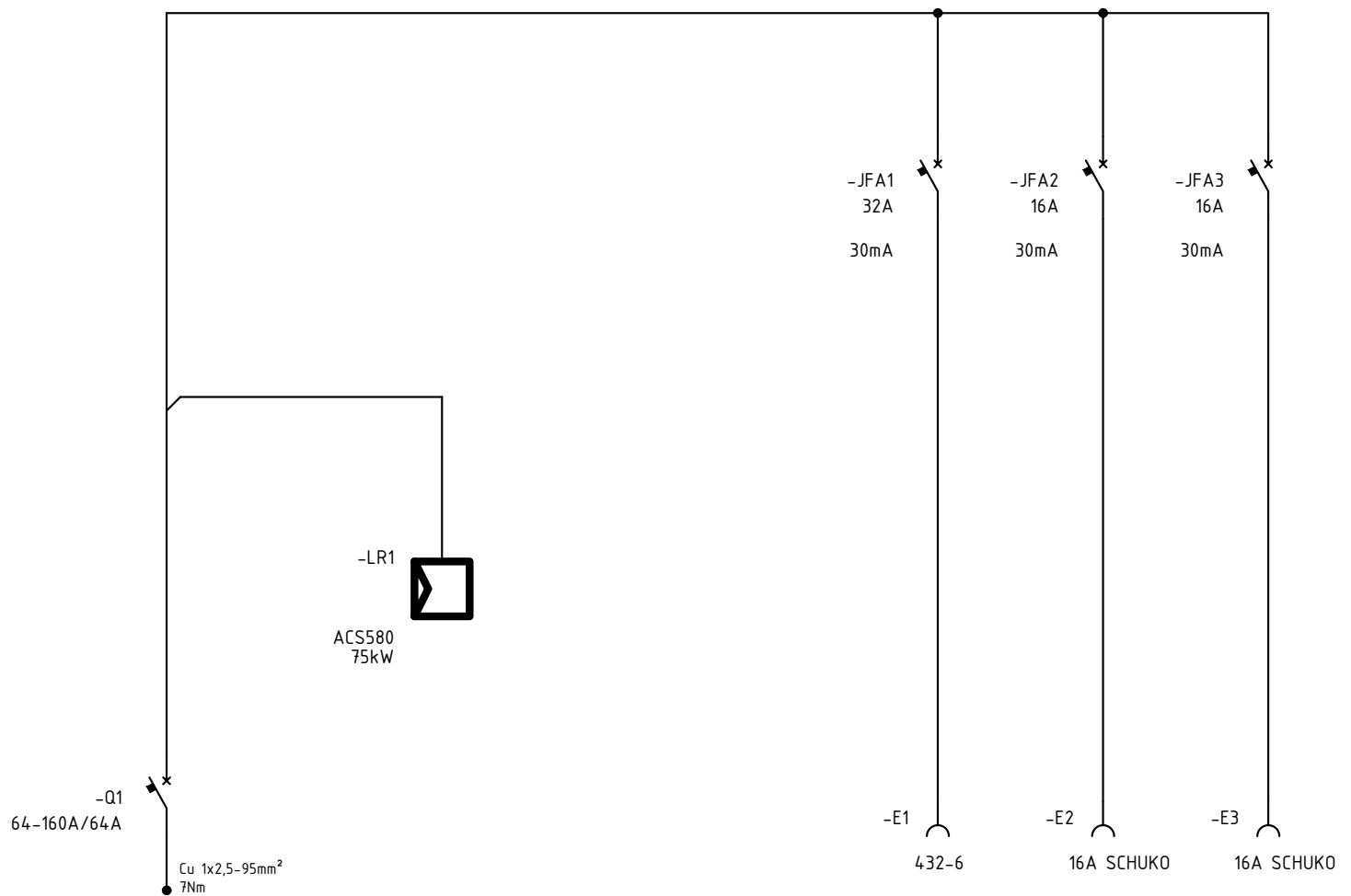
Enlinjeskjema
