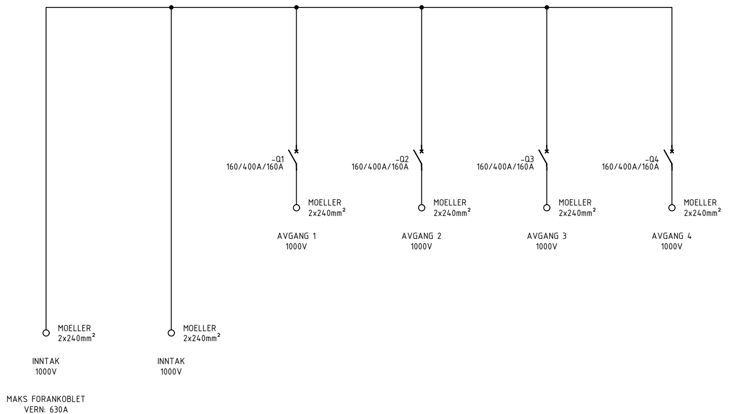
Enlinjeskjema
